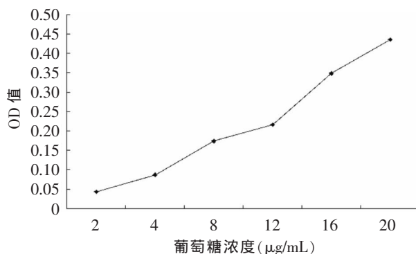
图 1 黑木耳多糖标准曲线
